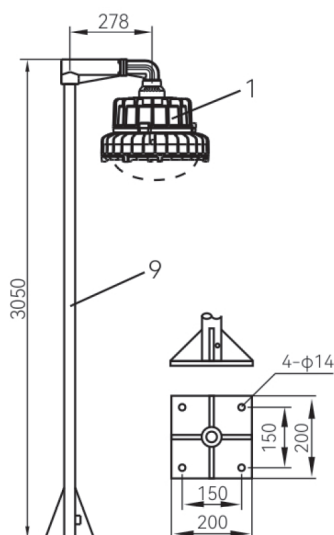
法兰式 (F1)
