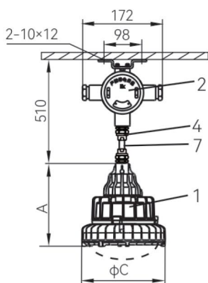
吊杆式(G)
