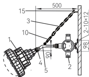
壁式(B1)30°
