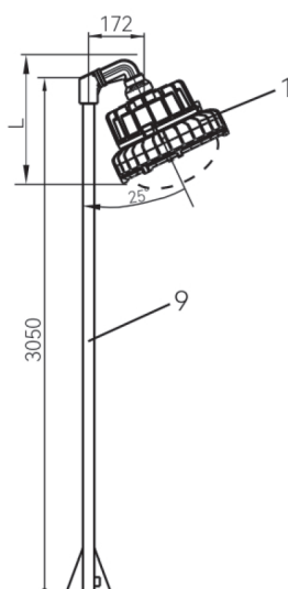
法兰式 (F2)
