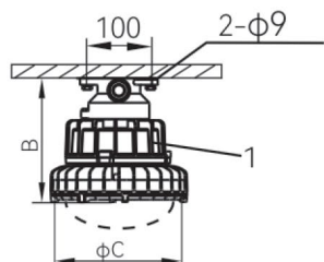
吸顶式 (X)
