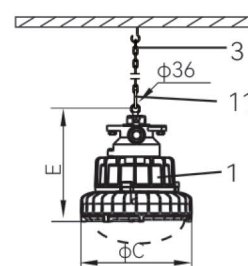
吊链式(D3)
