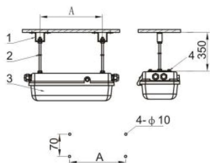
吊杆式 (G)
