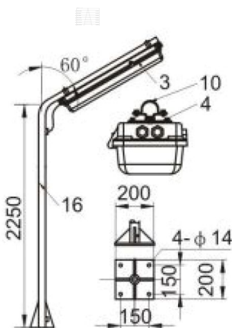
法兰式 (F)
