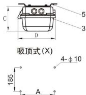
吸顶式 (X)
