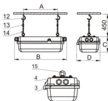
吊链式 (D)
