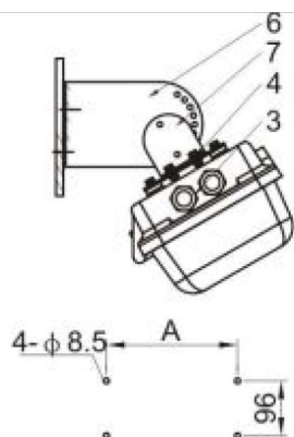
支架式 (Z)
