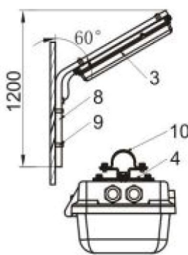
壁式 (B)
