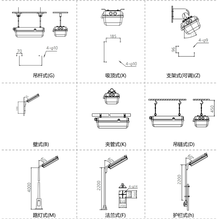
B-安装图
