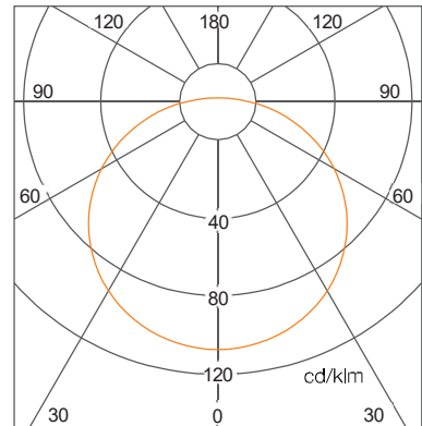
灯具配光曲线
